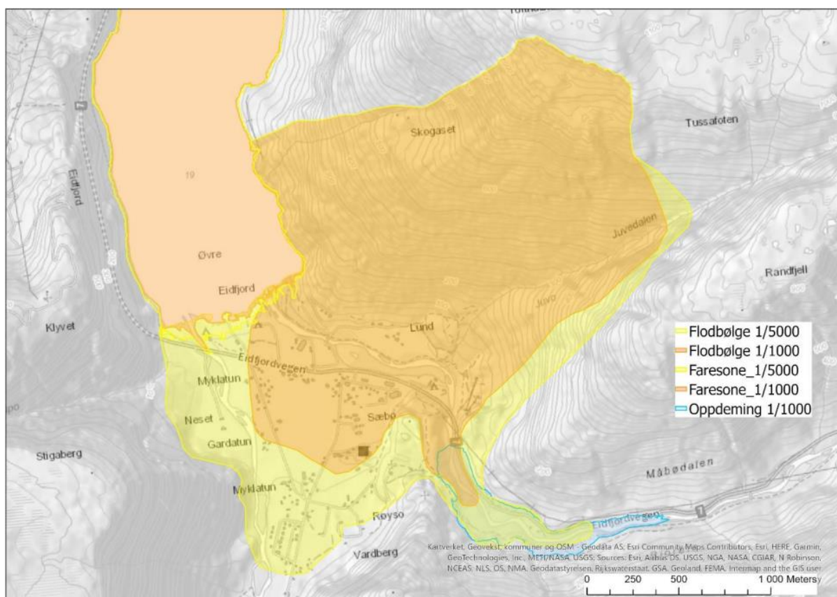
Figur 4 - Illustrasjon av faresonar ved ras frå Tussafoten. Henta frå NVE10.03.22.
