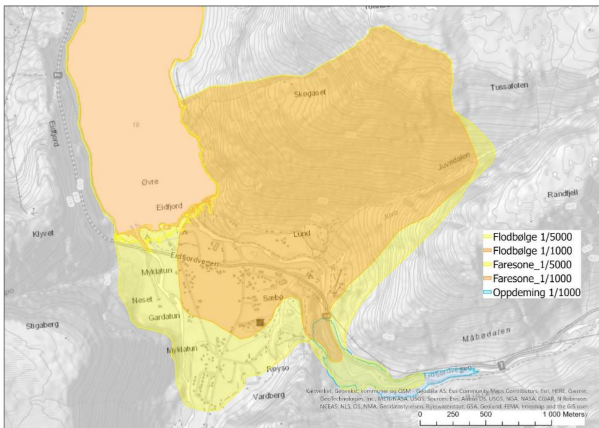
Figur 3 - Illustrasjon av faresonar ved ras frå Tussafoten. Henta frå NVE10.03.22.
