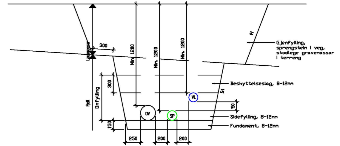
TYPISK GRØFTESNITT. Vatn-, spillvatn- og overvassledning
