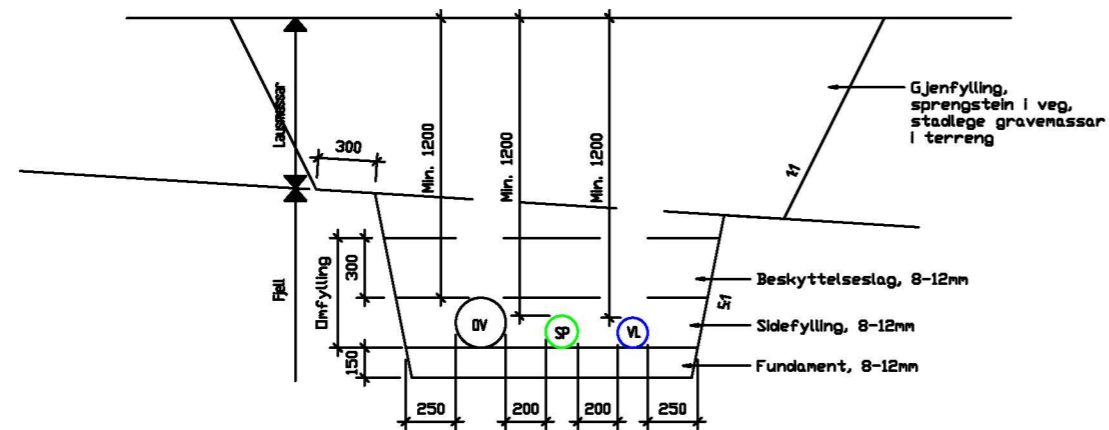
TYPISK GRØFTESNITT. Vatn-, spillvatn- og overvassledning
