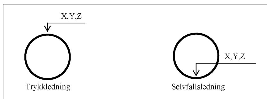
Figur 1. Måling av ledningshøyde.
