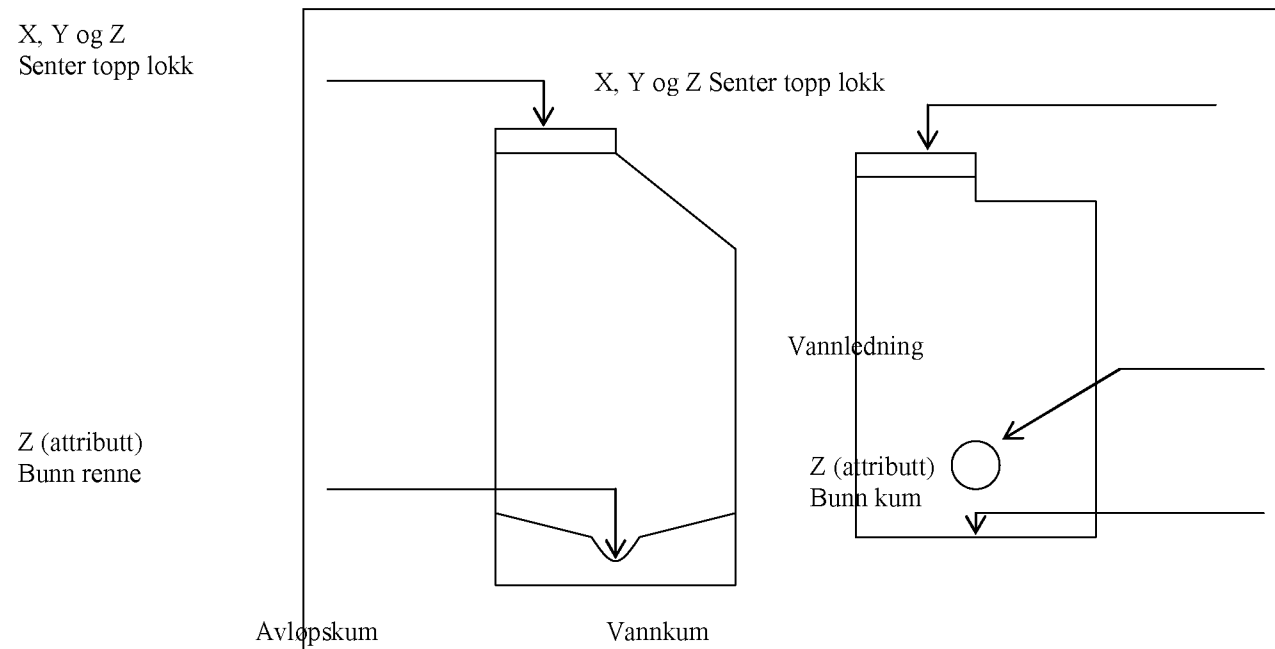
Figur 2. Innmåling av avløpskum og vannkum (snitt).
