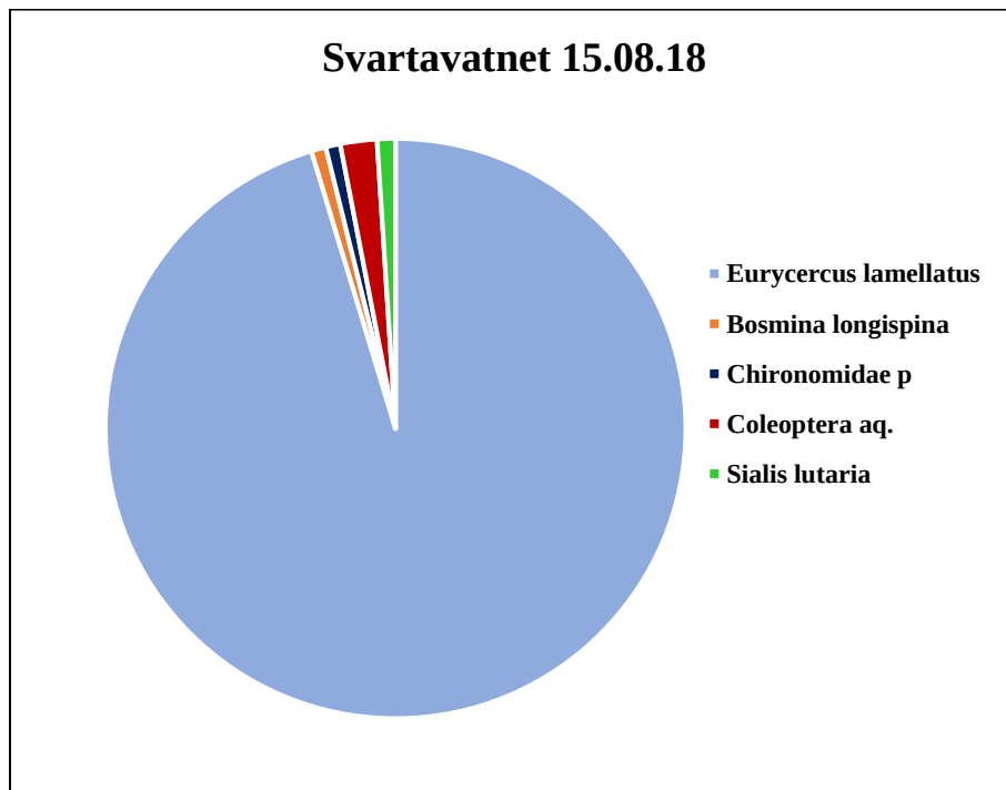
Figur 13. Sammensetning av mageinnhold fra aure i tatt på en garnserie i Svartavatnet 15. august 2018.
