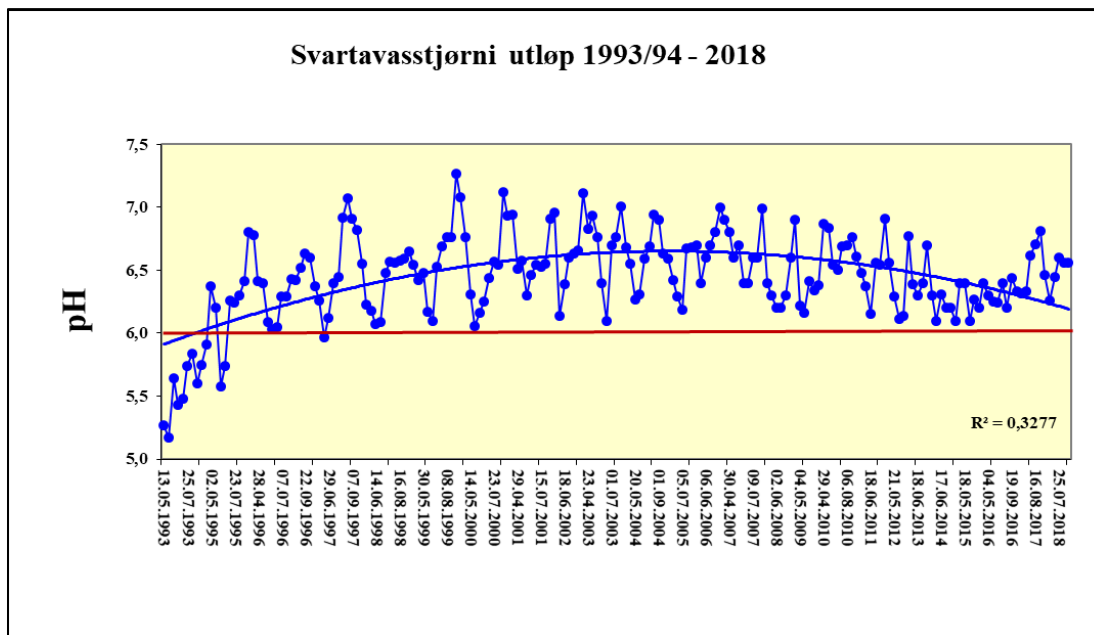
Figur 2. pH i utløpet av Svartavasstjørni i perioden 1993 – 2018.
