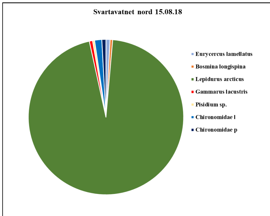
Figur 14. Sammensetning av mageinnhold fra aure tatt i Svartavatnet nord 15. august 2018.
