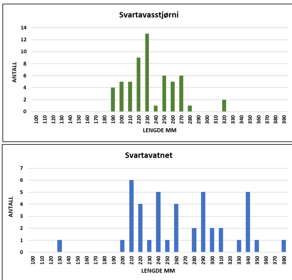
Figur 10. Lengdefordeling av aure i fangstene fra Svartavatnet og Svartavasstjørni i august 2018.
