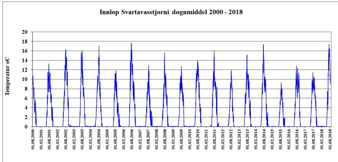
Figur 6. Vanntemperatur fra innløp Svartavasstjørni presentert som døgnmiddel 2000 – 2018.
