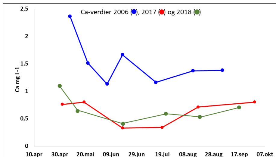
Figur14. Målte kalsiumverdier fra utløpet av Svartavasstjørni gjennom sesongene 2006 (●), 2017 (●) og 2018 (●).
