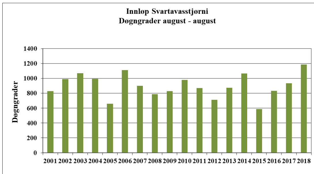
Figur 7. Antall døgngader fra august til august i innløp Svartavasstjørni 2000/01 – 2017/18.
